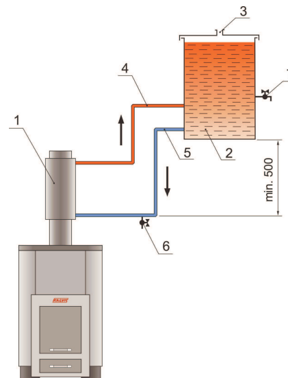
Рис. 6 Рекомендуемая схема подсоединения открытой емкости нагрева воды:
